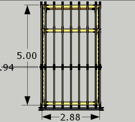
Plan 1:100
